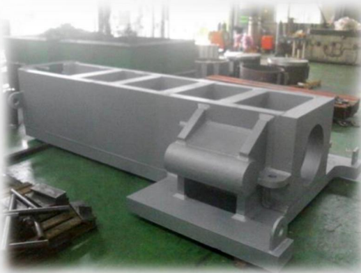
ロールテーブル 組立 ( Roller Table ASS'Y )
