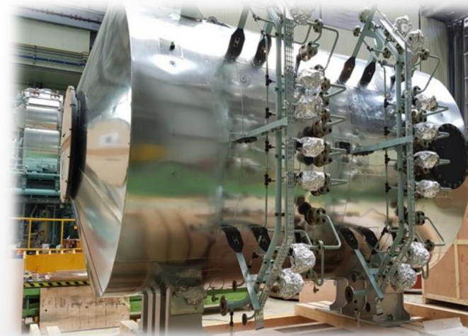
船舶エンジン排気ガス浄化装置_2 HP-SCR (Selective Catalytic Reduction)
