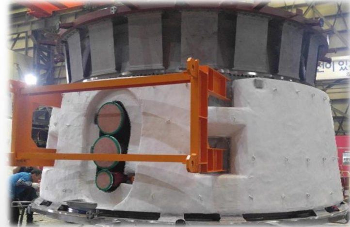
MHPS排気 マニホルド 保温-2 MHPS Exhaust Manifold Insulation
